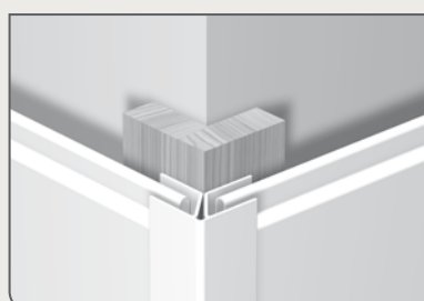
Knikhoekprofiel buitenhoek
